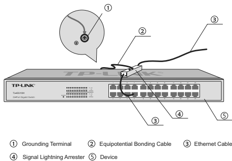
Figure 3-4 Equipotential Bonding
